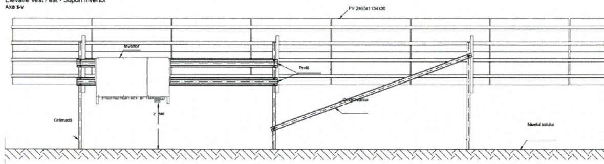
Figura 3. Desen indicativ - Detaliiu montaj inverter
