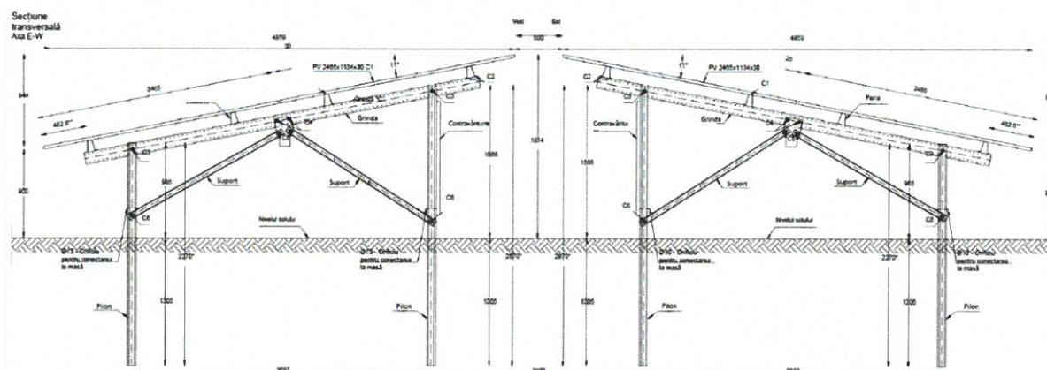
Figura 1. Desen indicativ - Detaliu structură fixă propusă (masă completă formată din 2 mese individuale)
